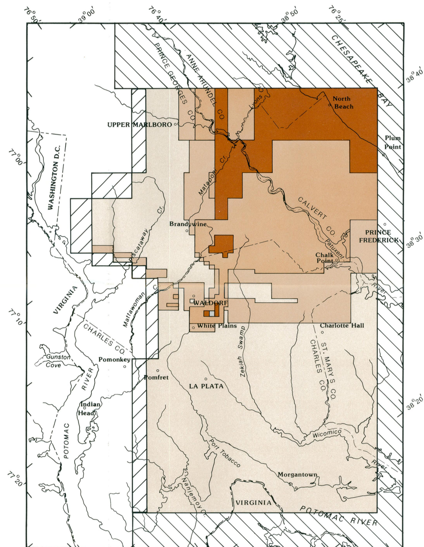
ST. CHARLES AQUIFER AND CORRELATIVE SANDS (D)
