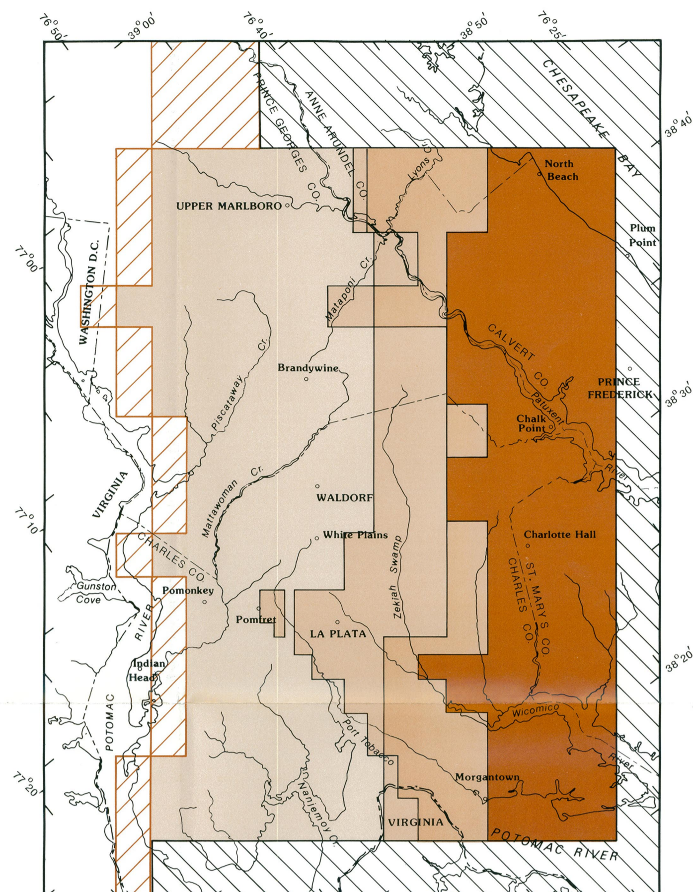
AQUIA AQUIFER (A)
